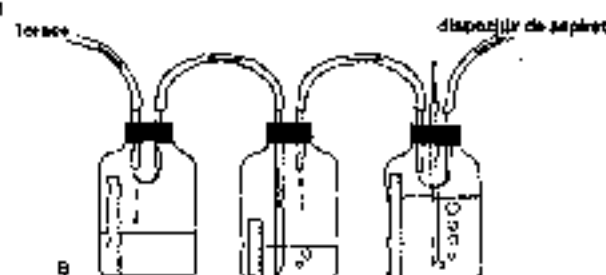
Fig. 7 – Sistem de drenaj cu trei flacoane
